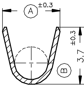
Secc. X-X'
