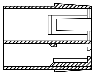
Secc. X-X'
