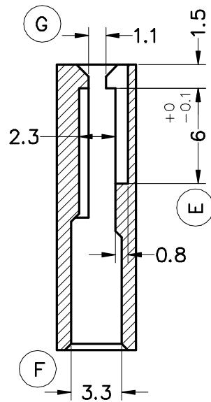
Sección A-A'
